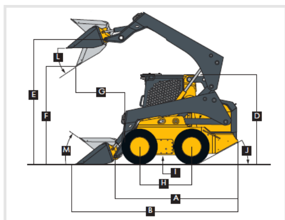
Dimensões principais (a)
